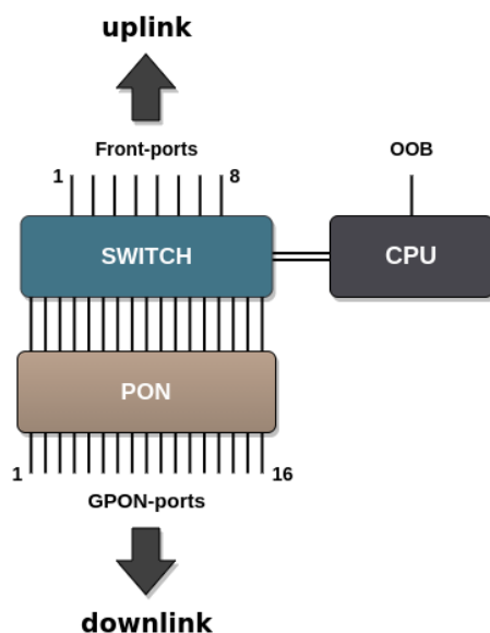
Рисунок 16 – Набор интерфейсов терминала
