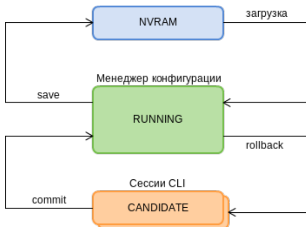
Рисунок 14 – Диаграмма жизненного цикла конфигурации терминала
