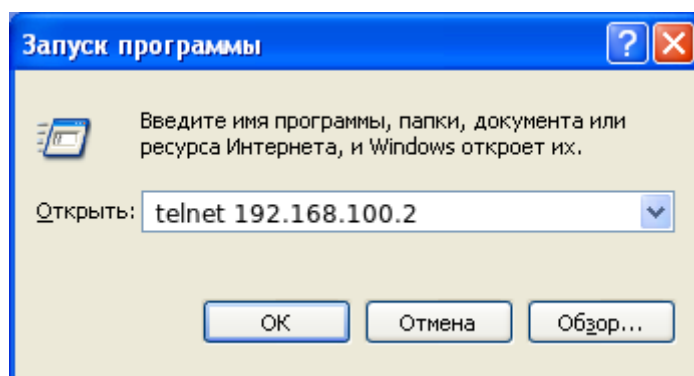
Рисунок 12 – Запуск клиента
