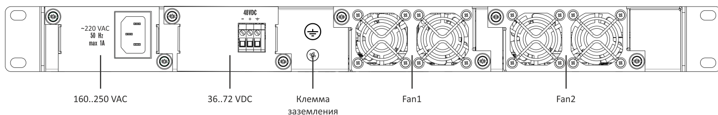
Рисунок 3 – Задняя панель станционного терминала LTP-16N/LTP-16NT
