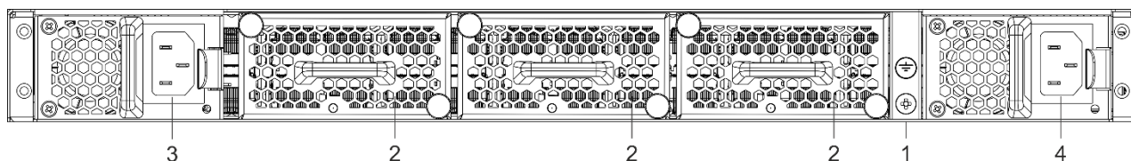
Рисунок 66 – Задняя панель MES5700-32
