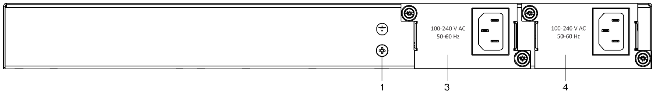
Рисунок 56 – Задняя панель MES3500I-24F
