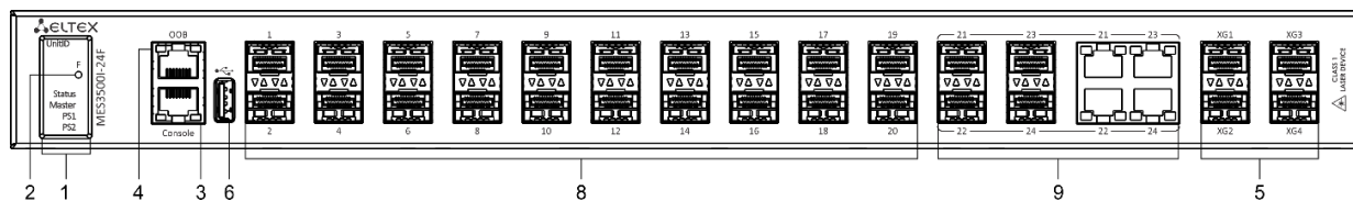
Рисунок 22 – Передняя панель MES3500I-24F
