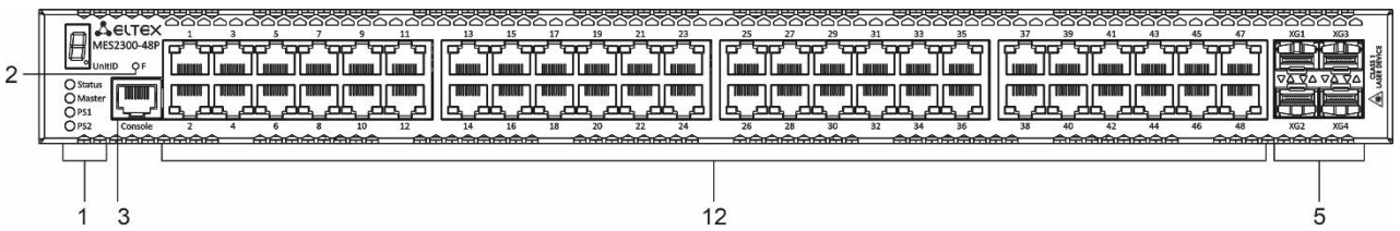
Рисунок 13 – Передняя панель MES2300B-48P
