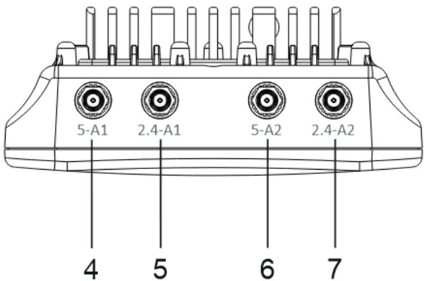
Рисунок 4 – Внешний вид верхней панели WOP-50L
