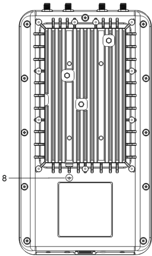
Рисунок 5 – Внешний вид задней панели WOP-50L
