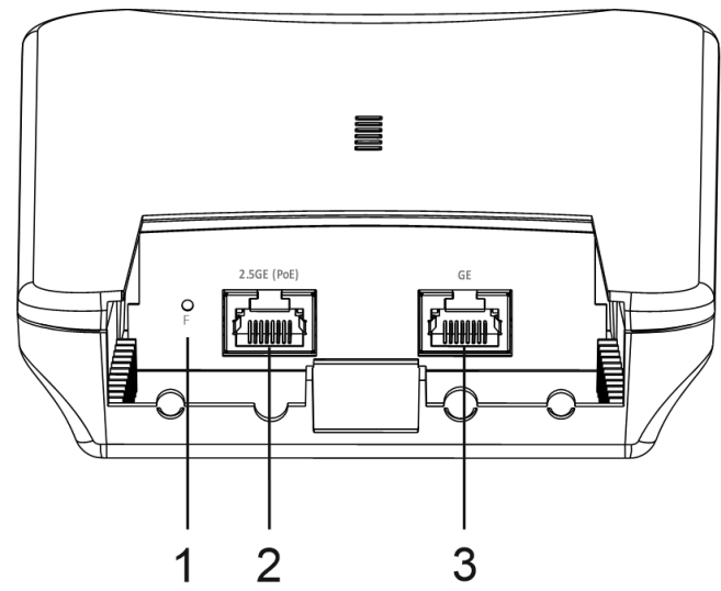
Рисунок 3 – Внешний вид нижней панели WOP-50L
