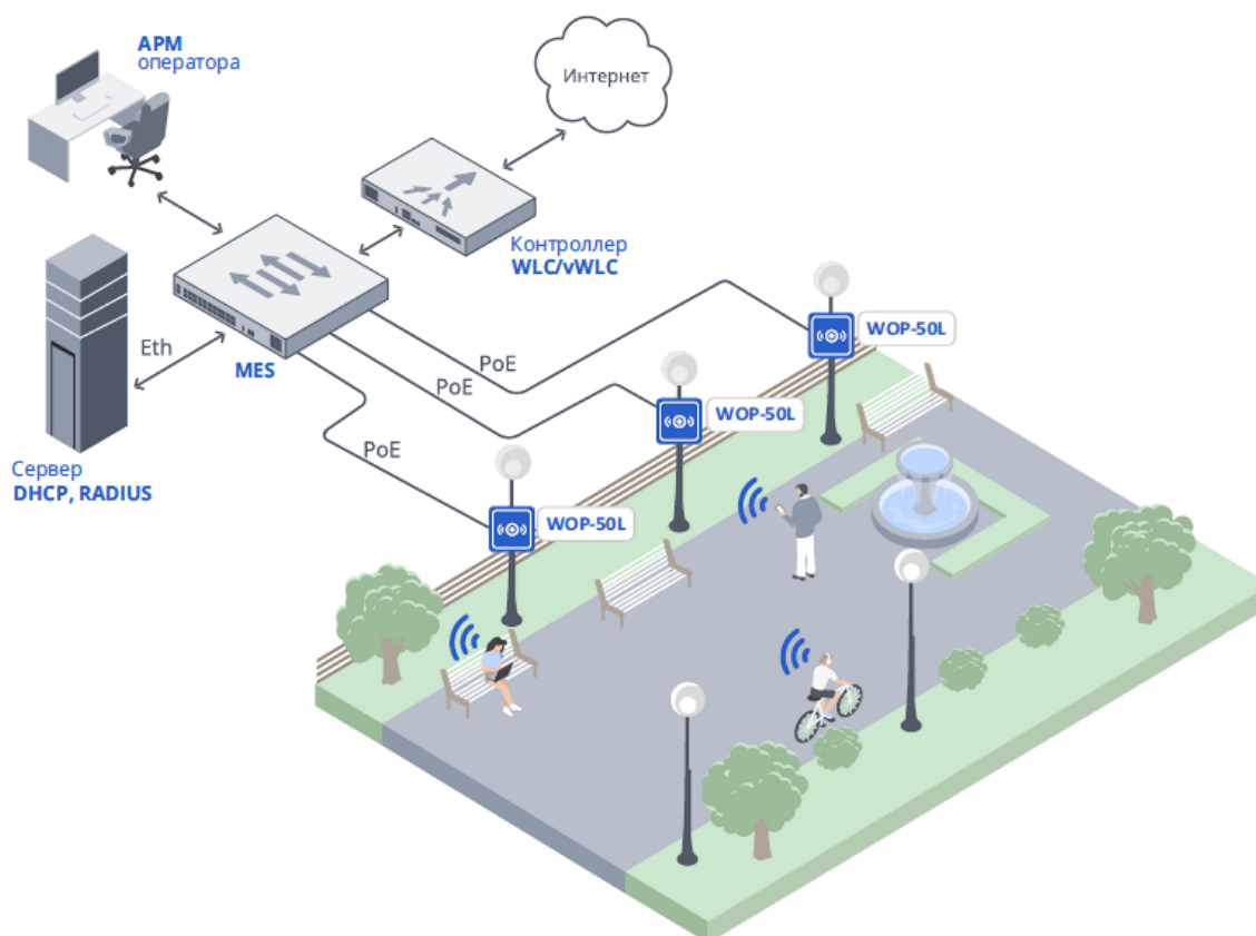
Рисунок 1 — Функциональная схема использования WOP-50L
