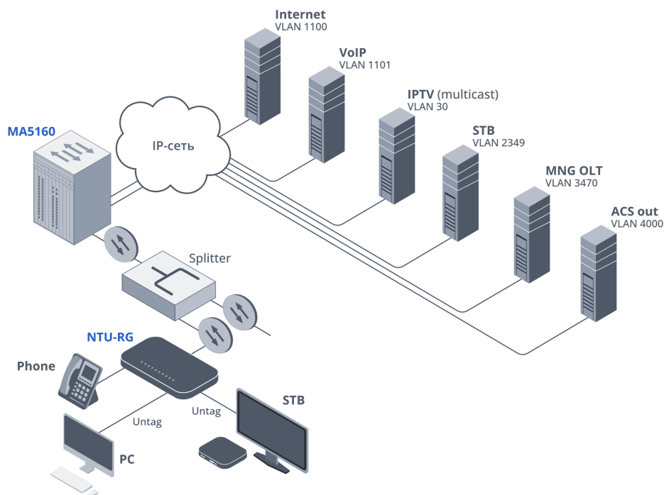
Рисунок 1 – Пример конфигурации сети
