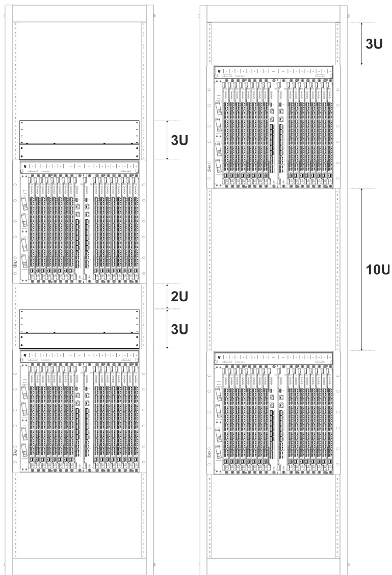
Рисунок 2 – Размещение MA5160 в стойке (с дефлектором MA5K16-FAND, без дефлектора)
