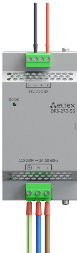
Рисунок 105 – Подключение питания к DRS-270-56
