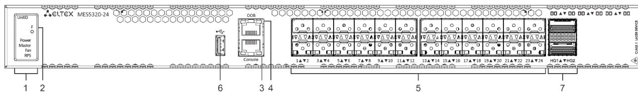
Рисунок 30 – Передняя панель MES5320-24
