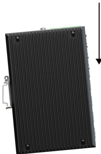
Рисунок 102 – Первый этап инсталляции MES на DIN-рейку
