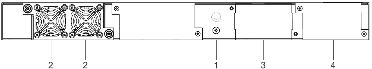
Рисунок 51 – Задняя панель MES3300-08F
