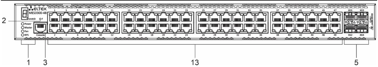
Рисунок 19 – Передняя панель MES3300-48
