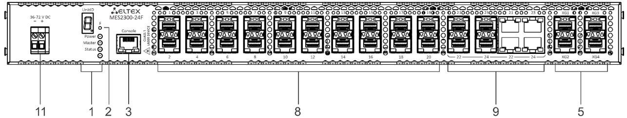
Рисунок 6 – Передняя панель MES2300D-24F
