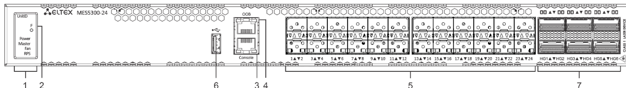
Рисунок 26 – Передняя панель MES5300-24
