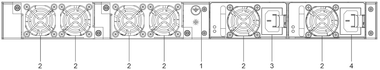
Рисунок 48 – Задняя панель MES2300-48P
