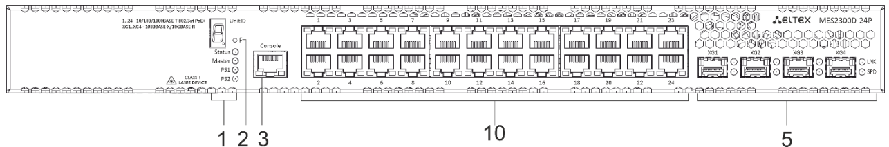
Рисунок 7 – Передняя панель MES2300D-24P
