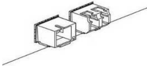
Рисунок 26 – Установка SFP-трансиверов
