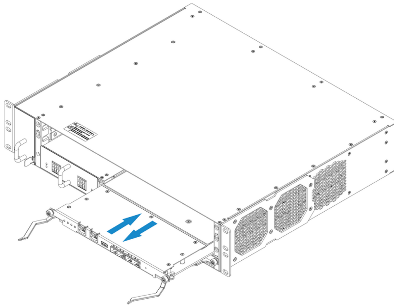
Рисунок 32 – Установка MA5K-FC16L в MA5020
