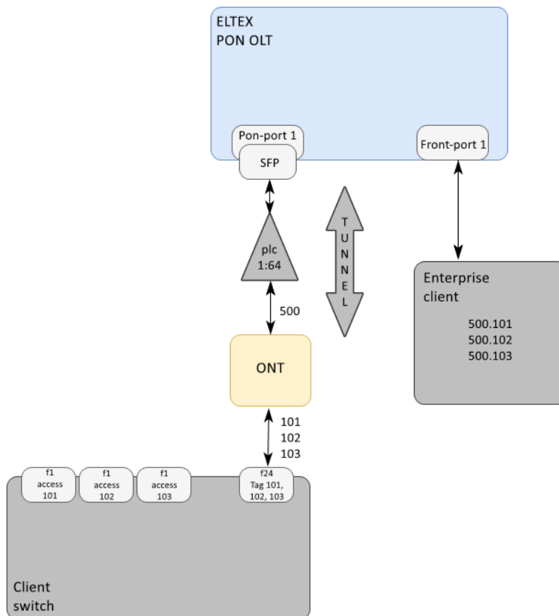
Рисунок 24 – Схема организации связи
