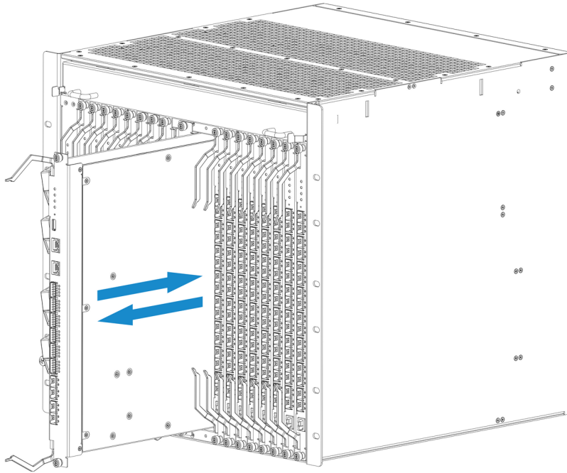
Рисунок 33 – Установка MA5K-FC64 в MA5160
