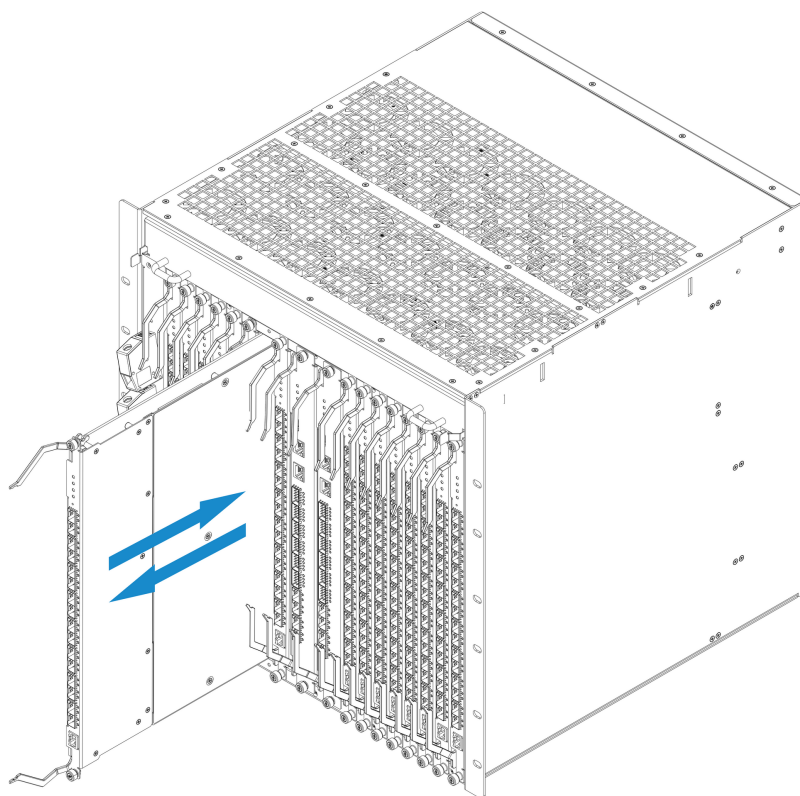
Рисунок 35 – Установка модулей интерфейсов PON в MA5160
