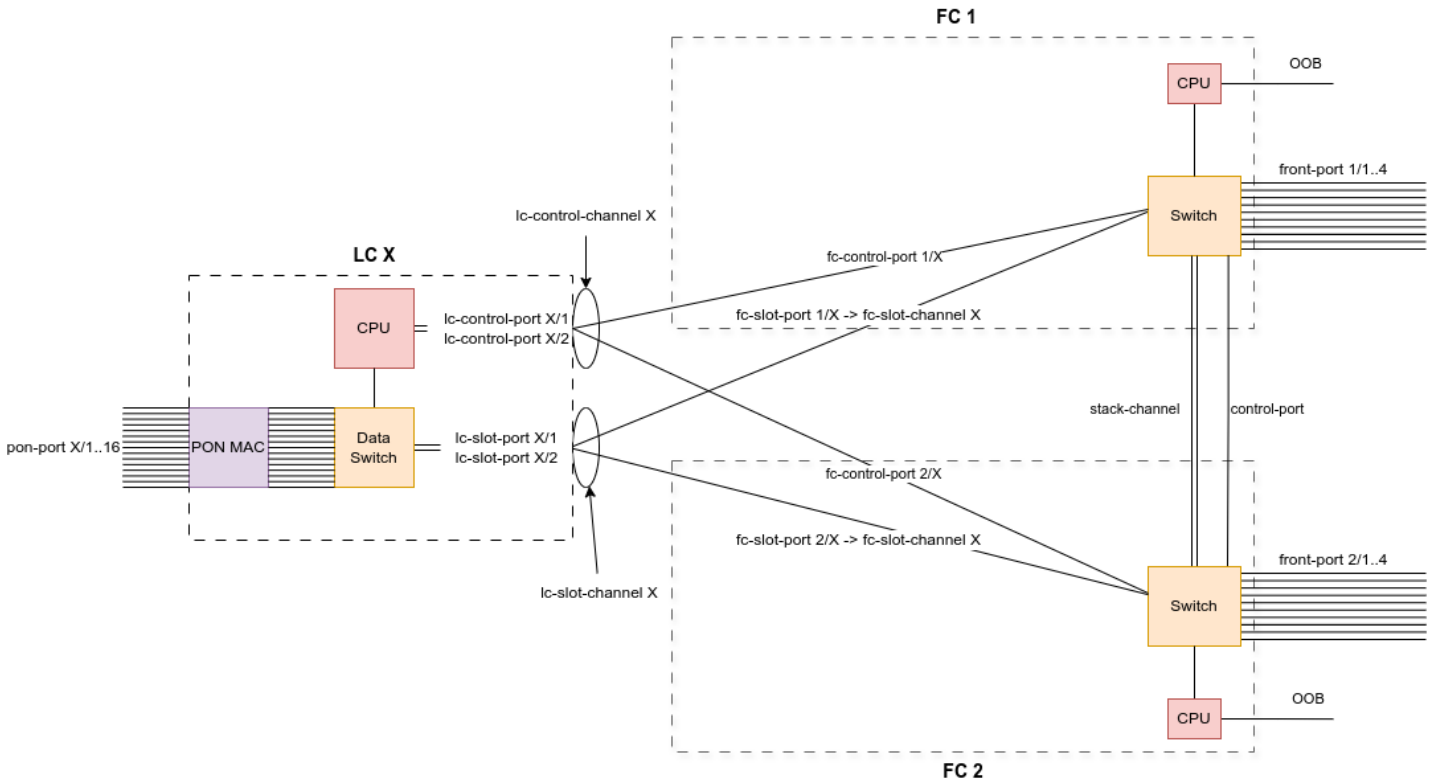
Рисунок 19а – Набор интерфейсов узла доступа MA5020
