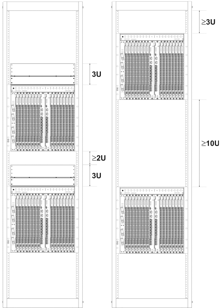
Рисунок 12 – Размещение MA5160 в стойке (с дефлектором MA5K16-FAND, без дефлектора)
