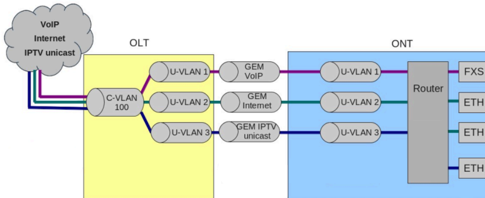
Рисунок 20 – Схема работы трафик-модели 1-to-1
