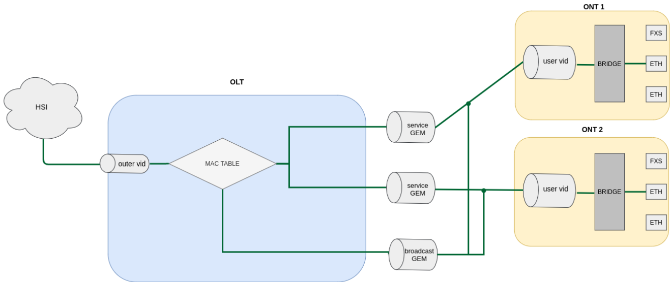
Рисунок 21 – Схема модели N-to-1
