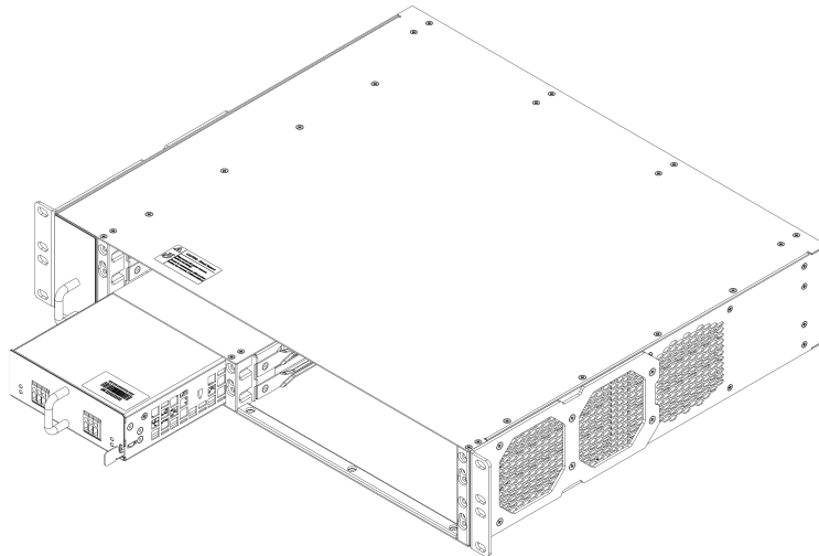
Рисунок 11 – Установка модуля питания MA5020
