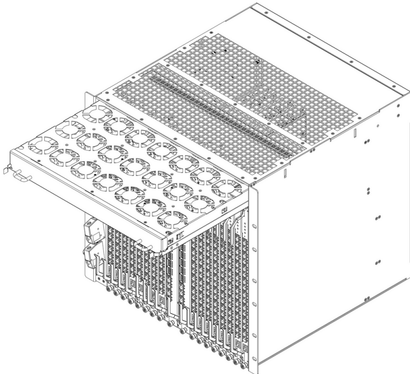
Рисунок 30 – Установка модуля вентиляции в MA5160
