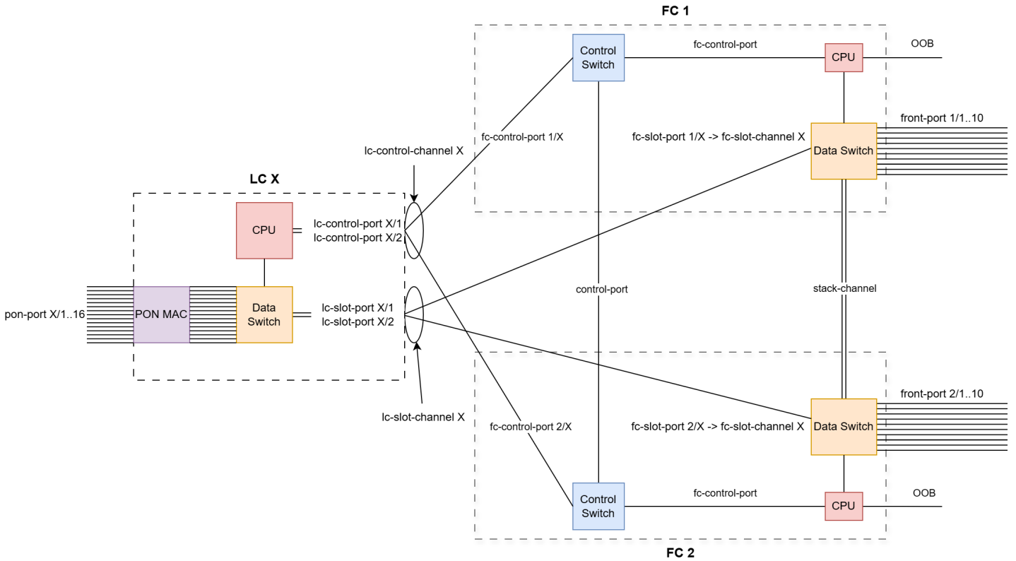
Рисунок 196 – Набор интерфейсов узла доступа MA5160
