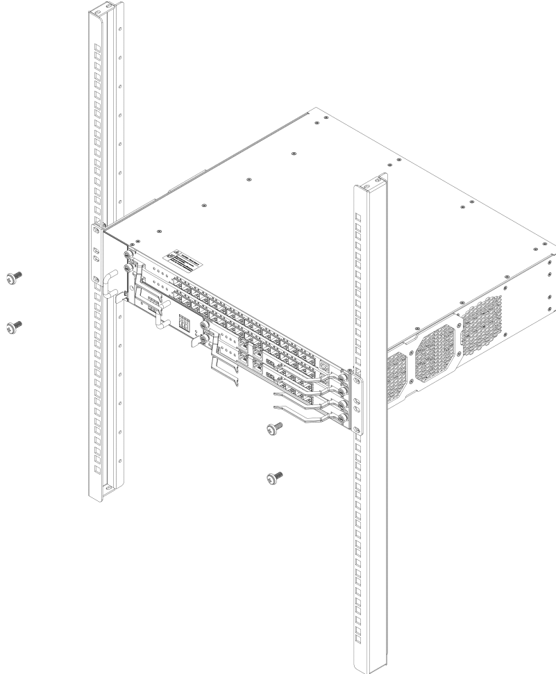
Рисунок 10 – Установка MA5020 в стойку
