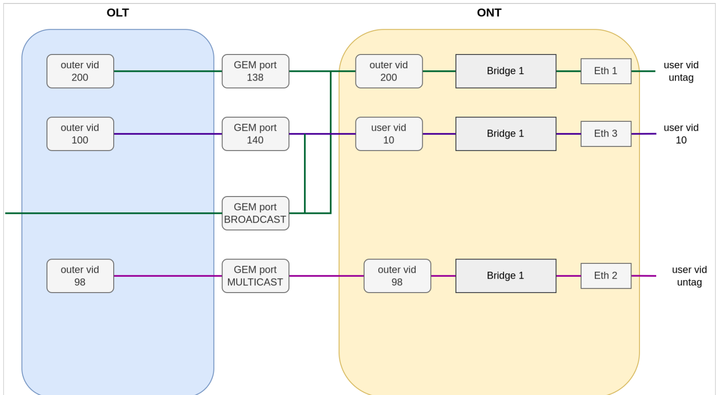
Рисунок 23 – Абстрактное представление тестовой конфигурации
