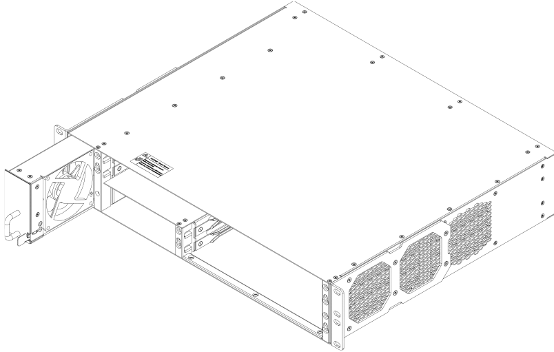
Рисунок 29 – Установка модуля вентиляции в MA5020
