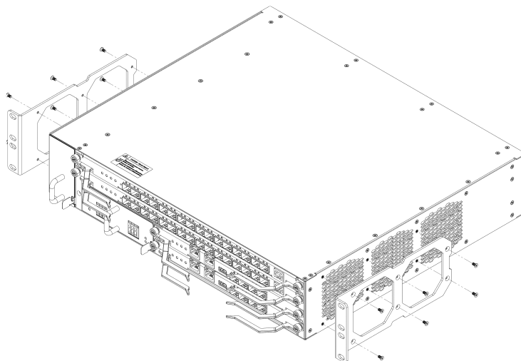
Рисунок 9 – Крепление кронштейнов MA5020
