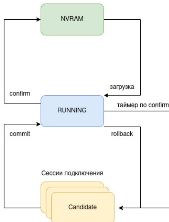
Рисунок 17 – Диаграмма жизненного цикла конфигурации узла доступа
