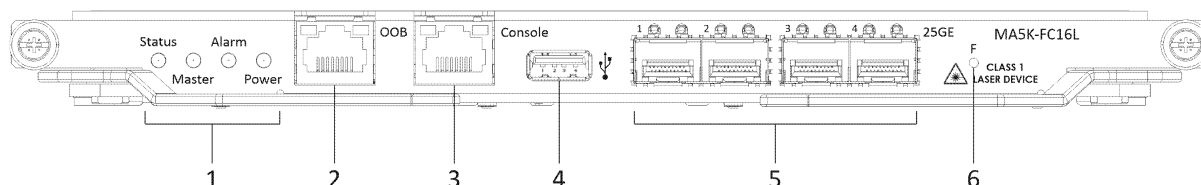
Рисунок 2 – Модуль управления и коммутации MA5K-FC16L
