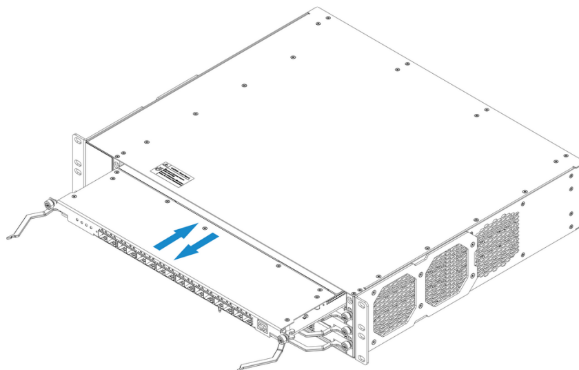
Рисунок 34 – Установка модулей интерфейсов PON в MA5020
