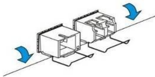
Рисунок 27 – Открытие защелки SFP-трансиверов
