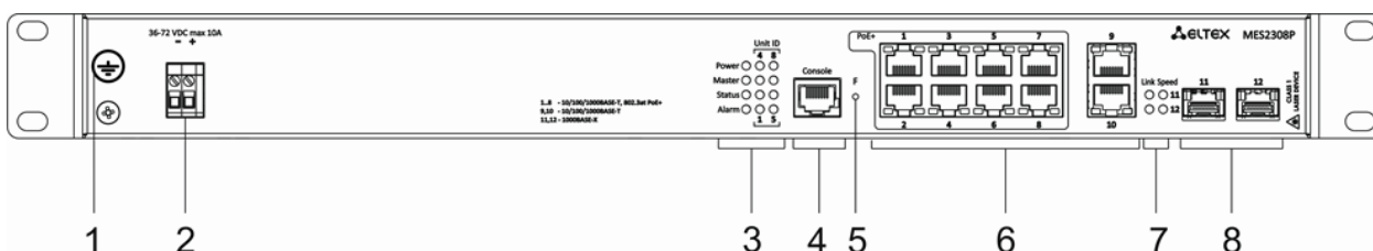
Рисунок 20 — Передняя панель MES2308P DC
