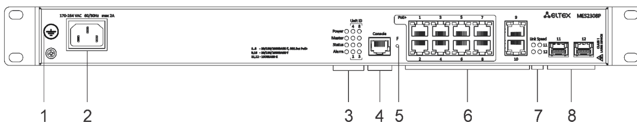
Рисунок 19 — Передняя панель MES2308P AC
