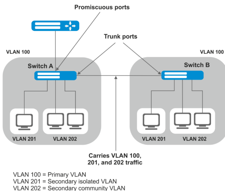
Рисунок 509 — Пример работы технологии Private VLAN
