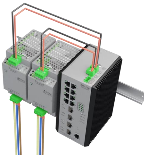
Рисунок 52 — Подключение коммутатора для питания от двух блоков DRS-270-56
