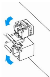
Рисунок 487 — Открытие защелки SFP-трансиверов
