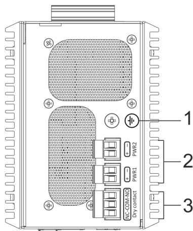
Рисунок 38 — Верхняя панель MES3508, MES3508P, MES3510P
