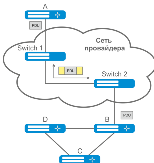
Рисунок 60 — Пример работы функции L2PT
