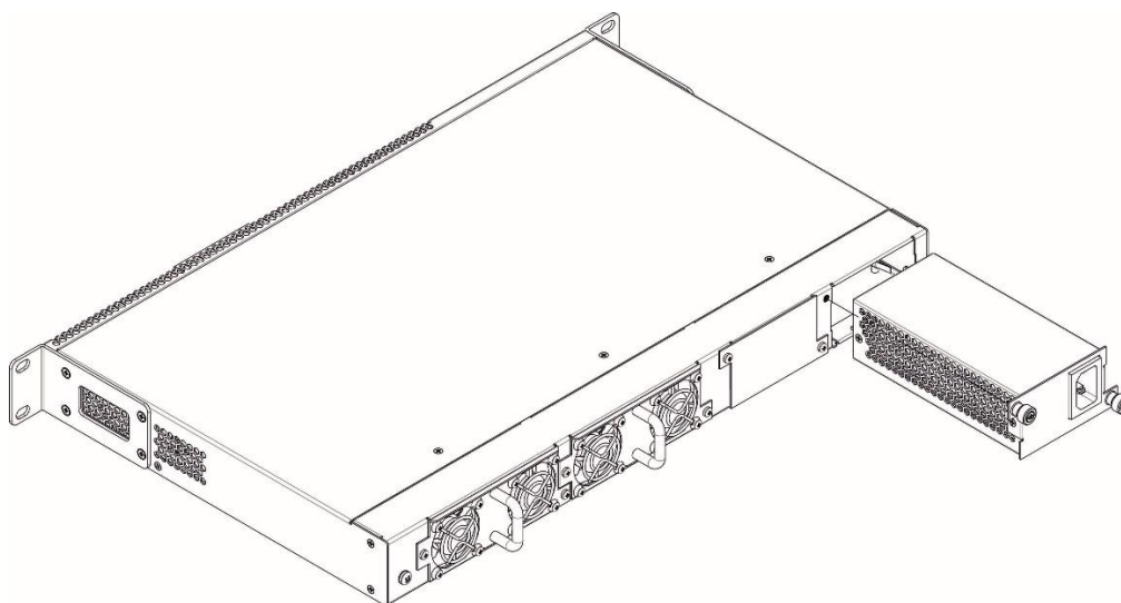
Рисунок 53 — Установка модулей питания
