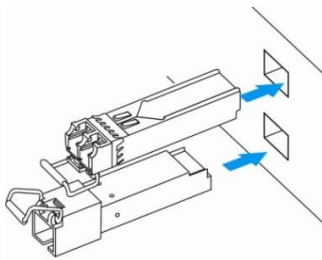
Рисунок 55 — Установка SFP-трансиверов
