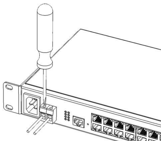
Рисунок 54 — Подключение АКБ к устройству
