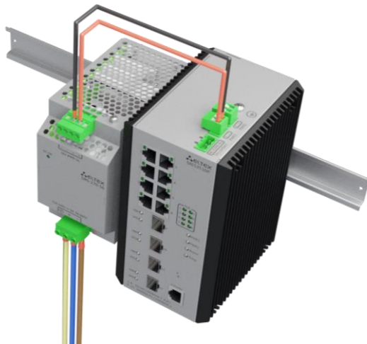
Рисунок 51 — Подключение коммутатора для питания от одного блока DRS-270-56
