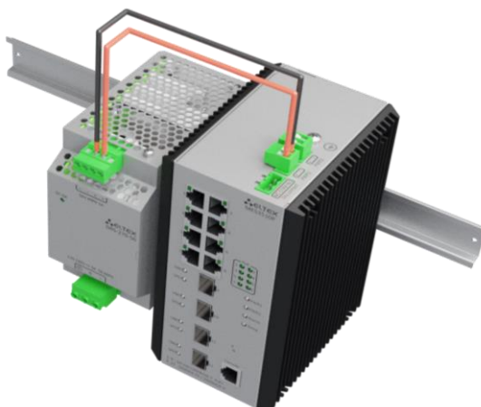
Рисунок 49 — Подключение питания коммутатора от DRS-270-56
