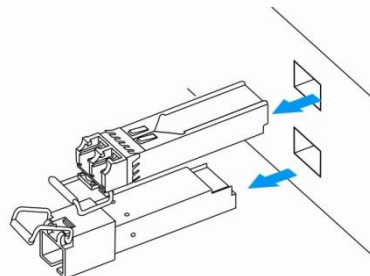
Рисунок 498 — Извлечение SFP-трансиверов
