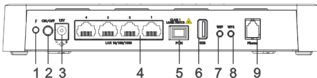
Рисунок 5 – Внешний вид задней панели NTU-RG-5521G-Wax
