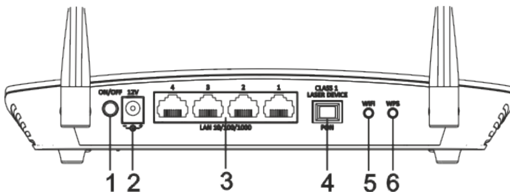
Рисунок 3 – Внешний вид задней панели NTU-RG-5520G-Wax rev.B
