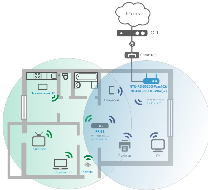
Рисунок 1 – Схема применения NTU-RG-5520G-Wax, NTU-RG-5520G-Wax rev.B, NTU-RG-5521G-Wax
