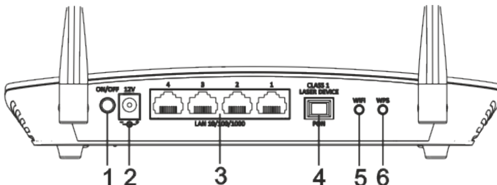
Рисунок 3 – Внешний вид задней панели NTU-RG-5520G-Wax rev.B
