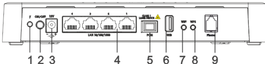
Рисунок 5 – Внешний вид задней панели NTU-RG-5521G-Wax
