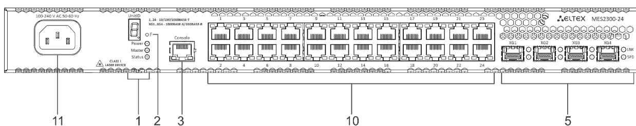
Рисунок 3 – Передняя панель MES2300-24
