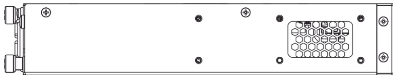
Рисунок 84 – Левая боковая панель MES5312
