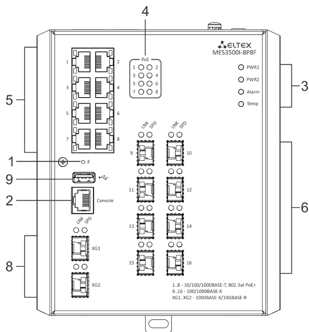
Рисунок 39 – Передняя панель MES3500I-8P8F
