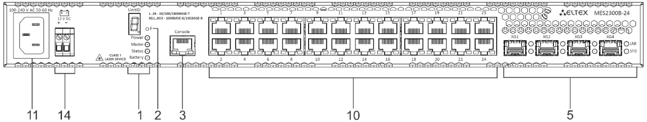
Рисунок 5 – Передняя панель MES2300B-24
