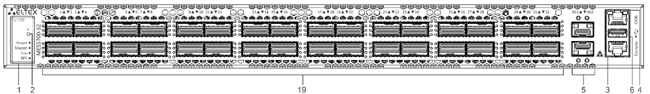
Рисунок 36 – Передняя панель MES5700-32
