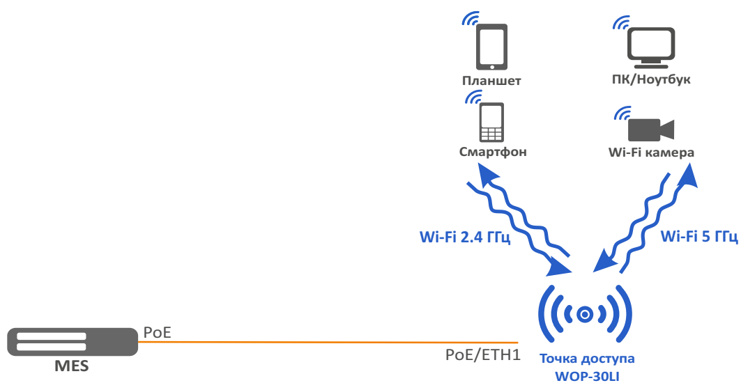
Использование точки доступа WOP-30LI с PoE-портом
