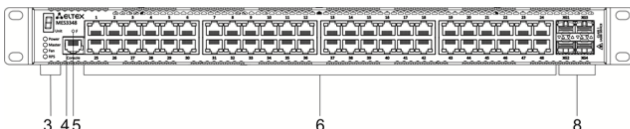
Рисунок 16 — Передняя панель MES3348
