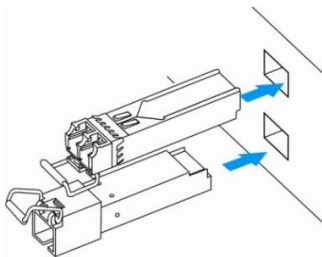
Рисунок 55 — Установка SFP-трансиверов
