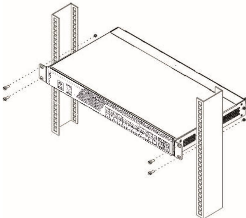
Рисунок 45 — Установка устройства в стойку
